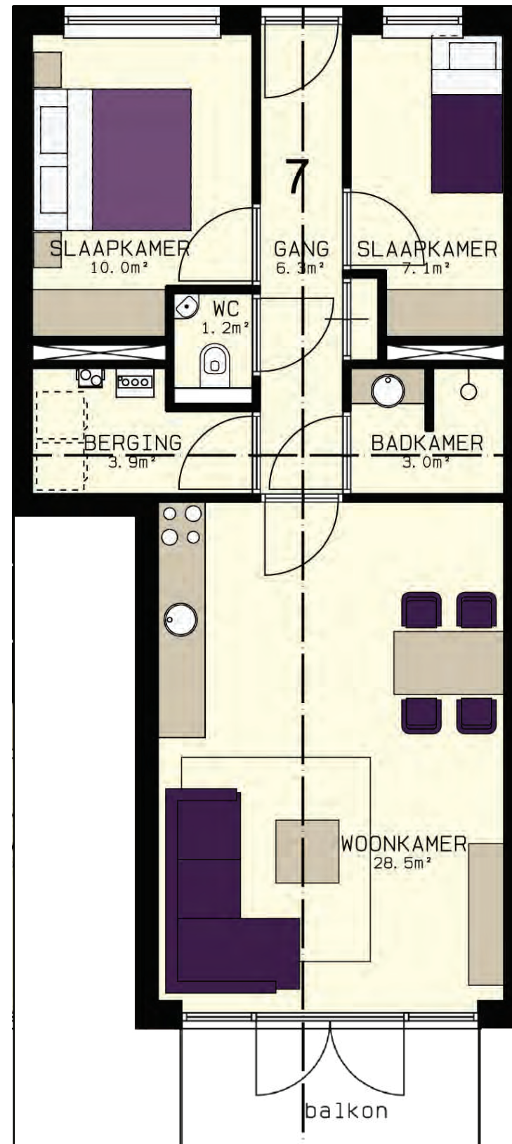
Appartement 7 - 1e verdieping - 66 m²
