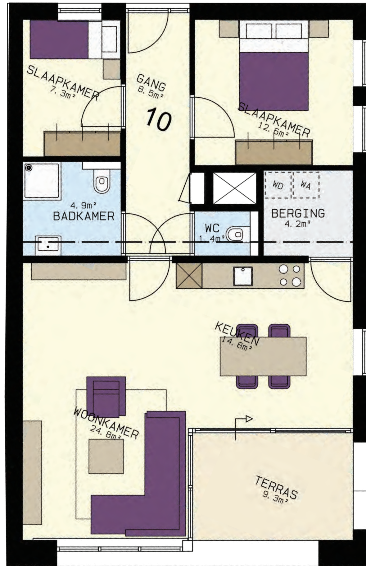
Appartement 10 - 1e verdieping - 84 m 2
